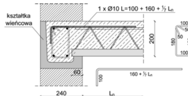
Rysunek 14. Zbrojenie wymienne
