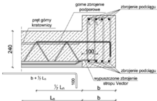
Rysunek 8. Oparcie płyt na nadciagu
