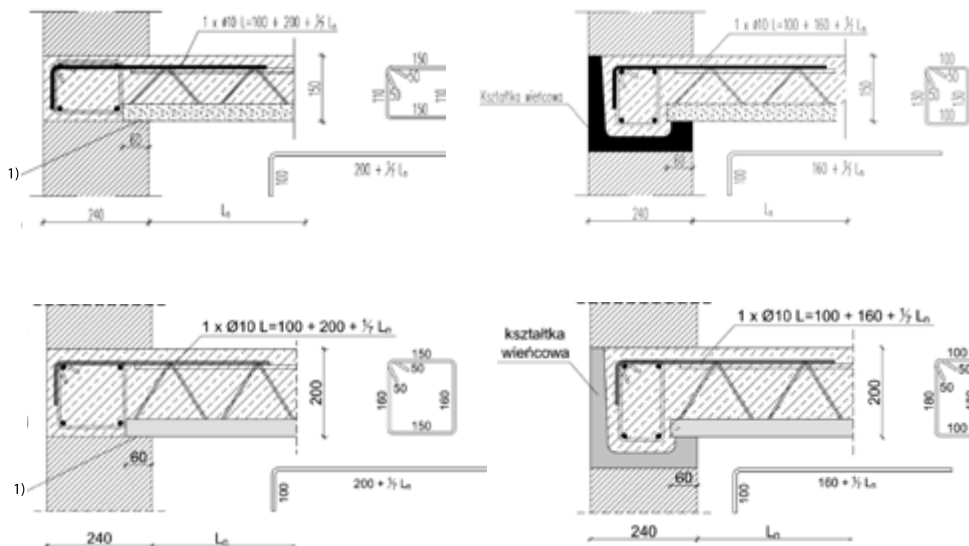
Rysunek 9. Oparcie pośrednie płyt na podporze skrajnej
