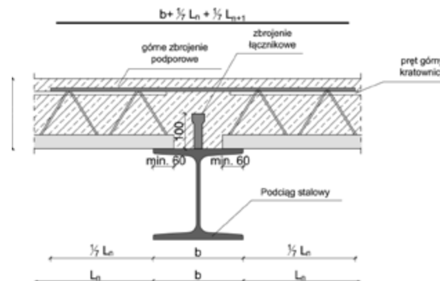
Rysunek 10. Oparcie stropu na belce stalowej
