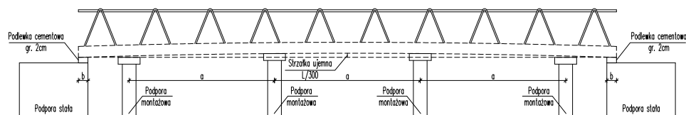
Rysunek 4. Sposób podparcia płyt na podporach
