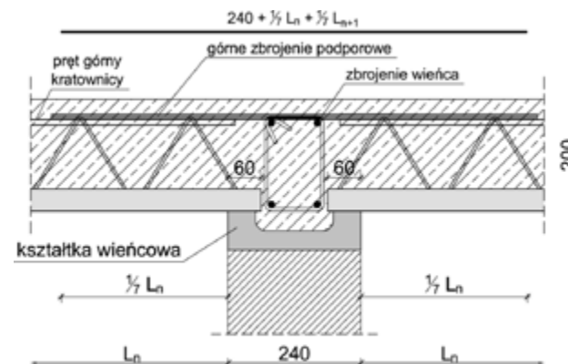
Rysunek 13. Dozbrojenie nadpodporowe
